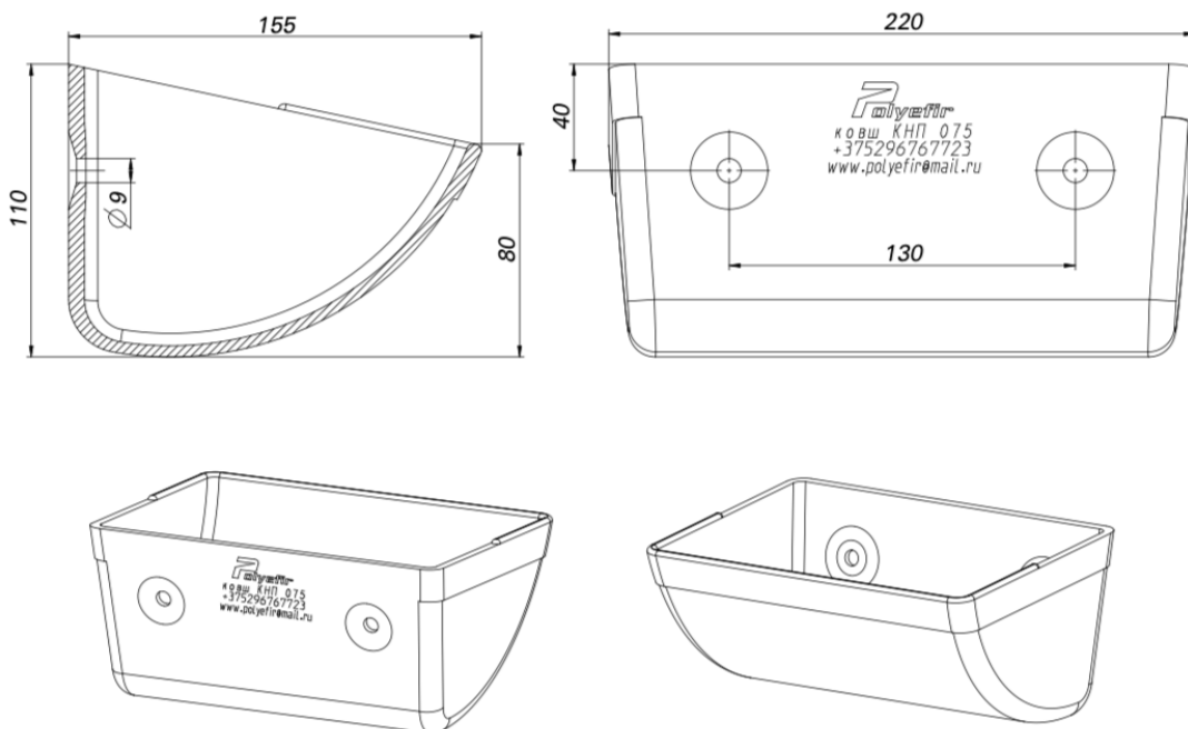
Ковш норийный КНП 075
