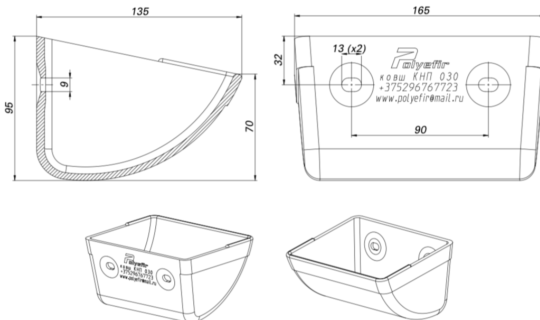
Ковш норийный КНП 030
